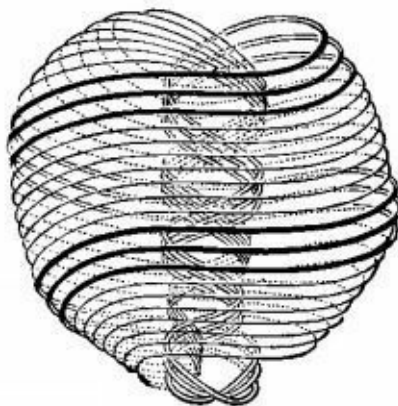
Рис. 7. Предельный физический атом.
