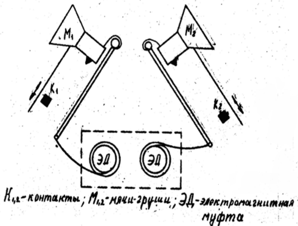
Рис.114 – Принципиальная электрическая и механическая схемы тренажера по борьбе дзюдо
