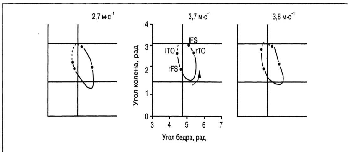
Рис. 110 – Диаграммы колено – бедро для трех человек с ампутацией ниже колена, бегущих со скоростью от 2,7 до 3,8 м*с (Епока, Miller, Burgess, 1982)
