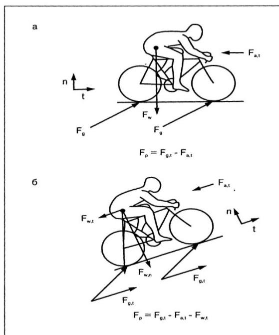
Рис. 105 – Диаграмма свободного тела системы велосипедиста.
